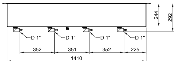
Boční
